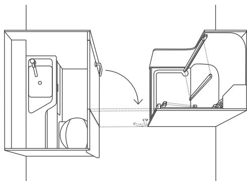
Baderommet i 700 MEG / 650 MEG
